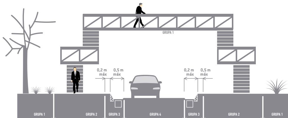
Usytuowanie włączów i wpustów wg Normy EN 124-2:2015
